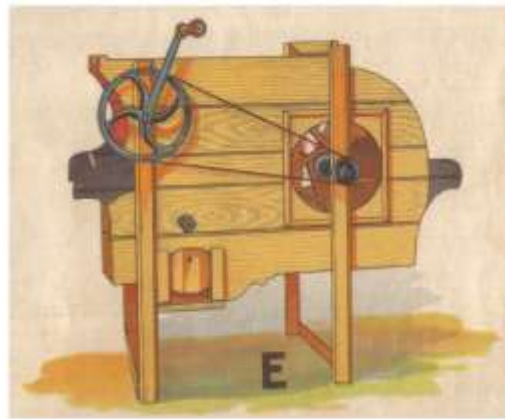
Schéma mlýnku na čištění obilí podle hmotnosti Ruční mlýnek (fukar) firmy V. Zima, Opočno
