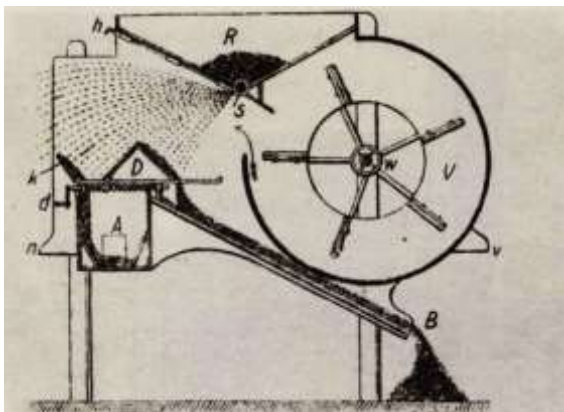
Schéma mlýnku na čištění obilí podle hmotnosti Ruční mlýnek (fukar) firmy V. Zima, Opočno
